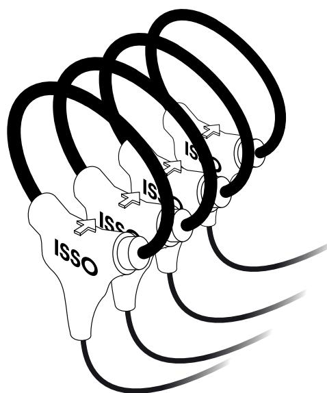
4 bobinas de Rogowski BR-Flex 40
